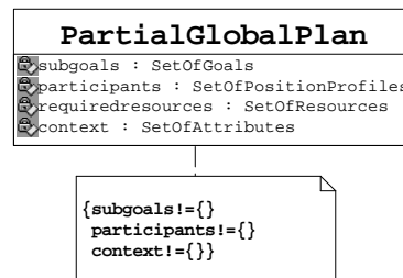
Fig. 11. Class PartialGlobalPlan
